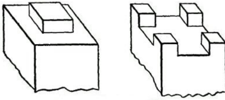
Fig. 293. Spur Tenon.
