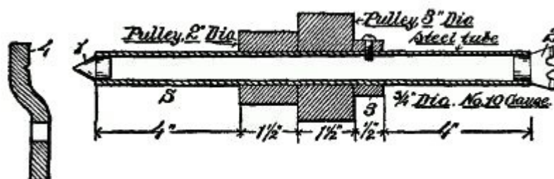
Fig. 244. Mandrel.
