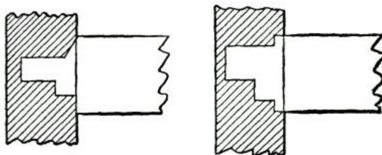
Fig. 299. Tusk Tenon.
