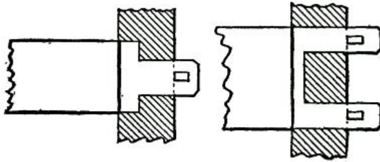
Fig. 300. Double Tusk Tenon.
