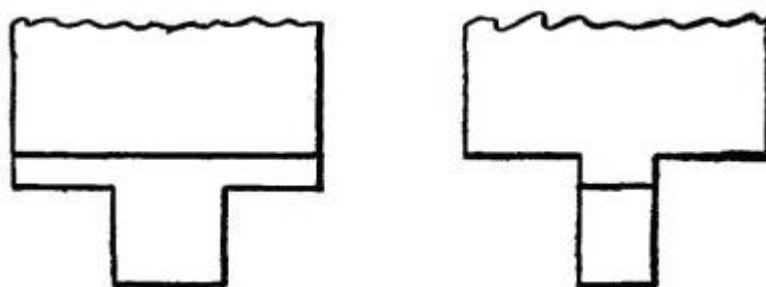
Fig. 298. Stub Tenon.
